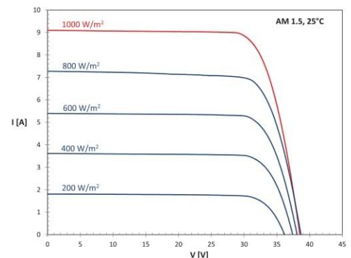
Charakterystyka prądowo-napięciowa
