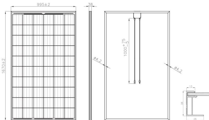
Wymiary modułu
